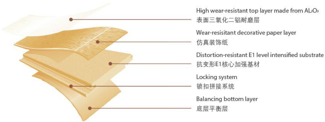
结构示意图
